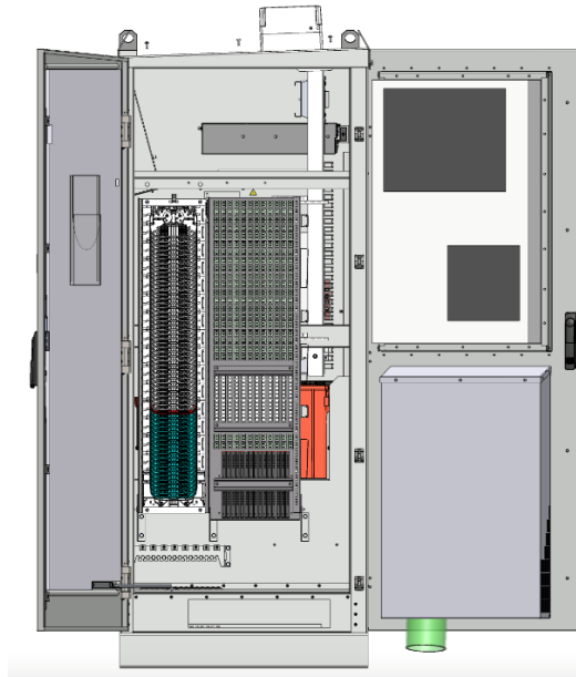
Sezione fibra ottica / permutazione
