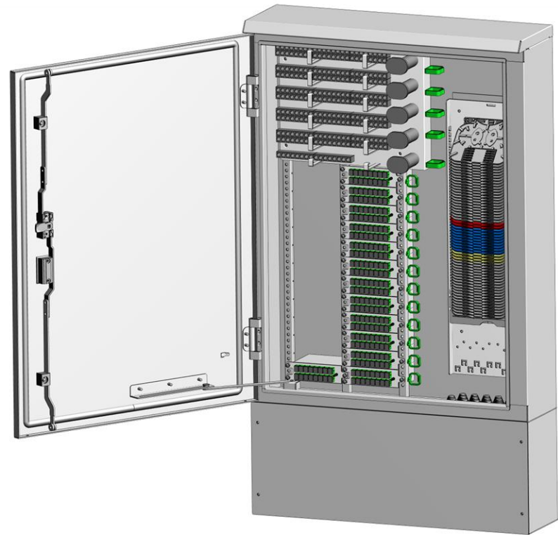
Cabinet PFS4 (Punto di Flessibilità Primario) Open Fiber
